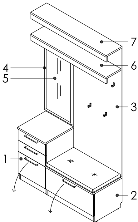
Композиция 1 ВШГ – 2269 x 1230 x 429
