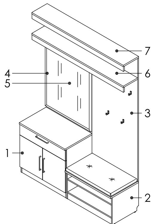
Композиция 4 ВШГ – 2269 x 1560 x 429
